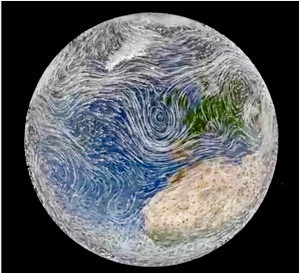
Structuur Zonnewarmte voorbeeld van luchtstroming over de Aarde
